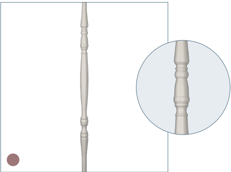
H-02 afwerking: voorgegrond, wit lengte: 970 mm doorsnede: Ø 22 mm gewicht: 0,35 kg afmeting sierwerk: 38 x 515 mm (bxh)
