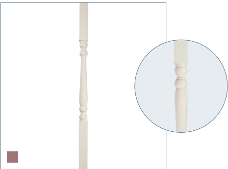
H-06 afwerking: voorgegrond, wit lengte: 970 mm doorsnede: 40 x 40 mm gewicht: 0,50 kg afmeting sierwerk: 40 x 376 mm (bxh)
