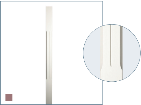
HB-03 afwerking: voorgegrond, wit lengte: 1.500 mm doorsnede: 90 x 90 mm gewicht: 5,2 kg afmeting sierwerk: 700 mm (bxh)
