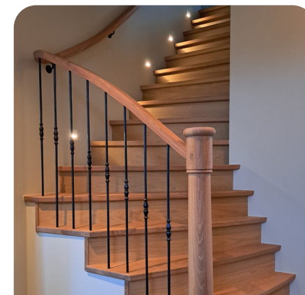
Trapspijl: S-22 Leuningdrager: LH-02
