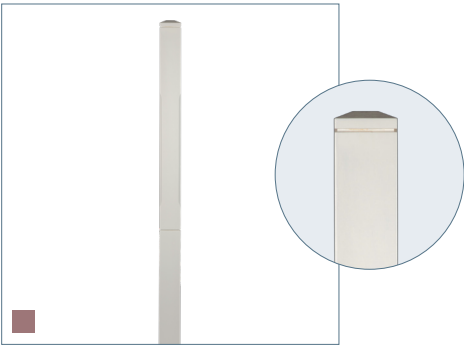
HB-04 afwerking: voorgegrond, wit lengte: 1.485 mm doorsnede: 91 x 91 mm gewicht: 5,9 kg lengte bewerking: 530 mm
