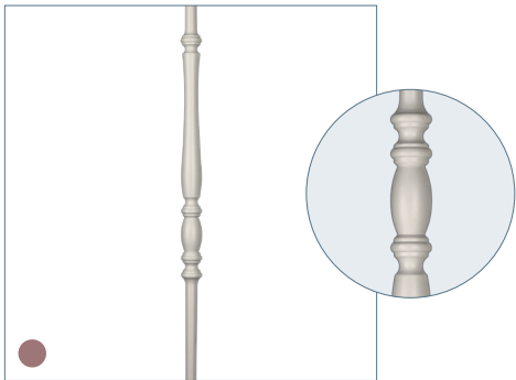
H-05 afwerking: voorgegrond, wit lengte: 970 mm doorsnede: Ø 22 mm gewicht: 0,36 kg afmeting sierwerk: 40 x 500 mm (bxh)
