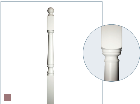
HB-01 afwerking: voorgegrond, wit lengte: 1.500 mm doorsnede: 90 x 90 mm gewicht: 4,7 kg afmeting sierwerk: 590 mm (bxh)
